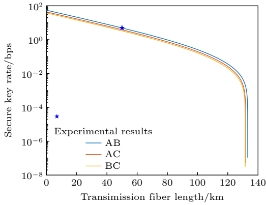
图 5 在超纠缠网络中 Alice, Bob 和 Charlie 之间的安全密钥速率随传输距离的变化
