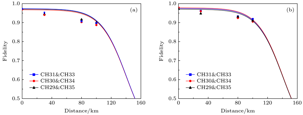
图 4 纠缠保真度与传输距离的关系 (a) time-bin 纠缠保真度与传输距离的关系; (b) 偏振纠缠保真度与传输距离的关系
